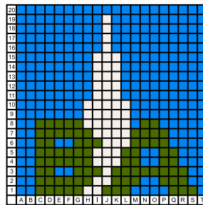
Plano Cartesiano
